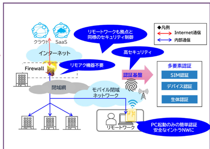
図 2:「S-NICS SIM MFA Plus」を使ったリモートアクセス構成概要
