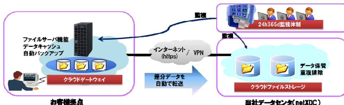
USiZE クラウドファイルサーバの構成図
